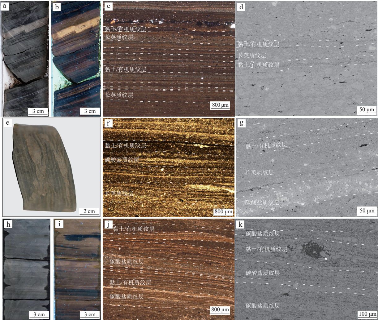
图 2 渤海湾盆地沧东凹陷孔店组二段不同纹层状页岩典型纹层结构显微照片
