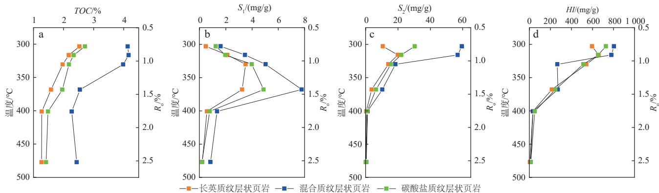
图5 渤海湾盆地沧东凹陷孔店组二段不同纹层状页岩有机地球化学特征
