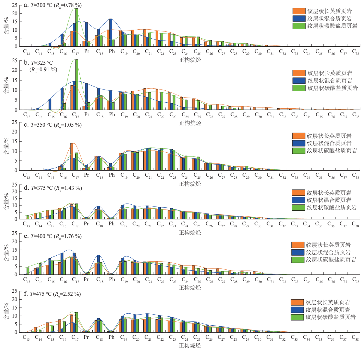
图13 渤海湾盆地沧东凹陷孔店组二段不同纹层状页岩在不同模拟温度下滞留油饱和烃组分含量分布柱状图
