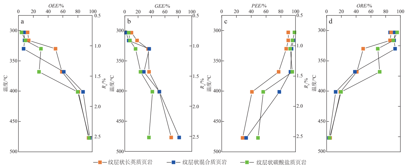
图11 渤海湾盆地沧东凹陷孔店组二段不同纹层状页岩生-排-滞效率随温度的变化
