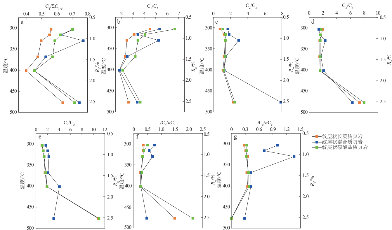
图12 渤海湾盆地沧东凹陷孔二段不同纹层状页岩气态饱和烃产物参数随温度的变化
