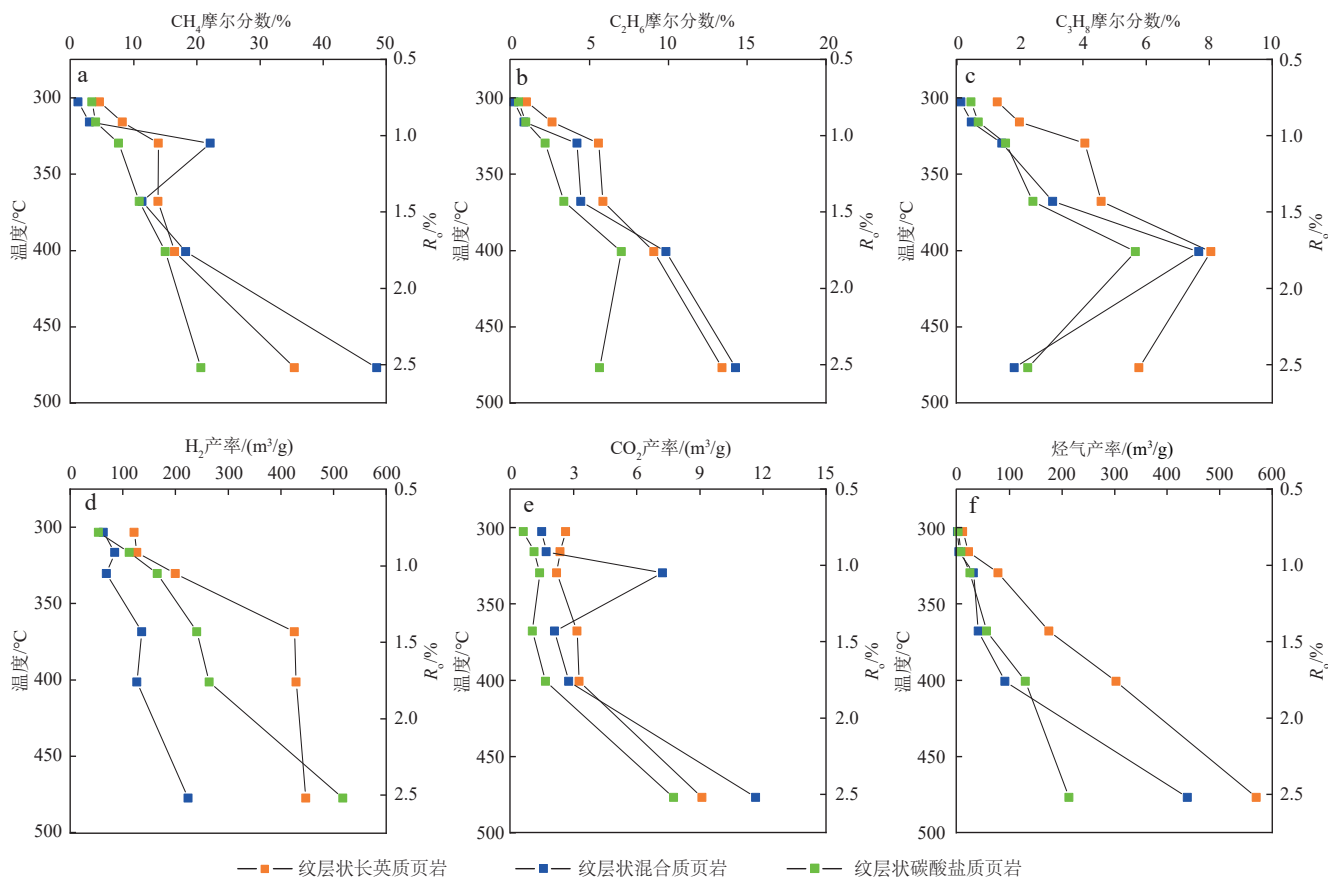
图8 渤海湾盆地沧东凹陷孔店组二段不同纹层状页岩气态产物产率与温度关系
