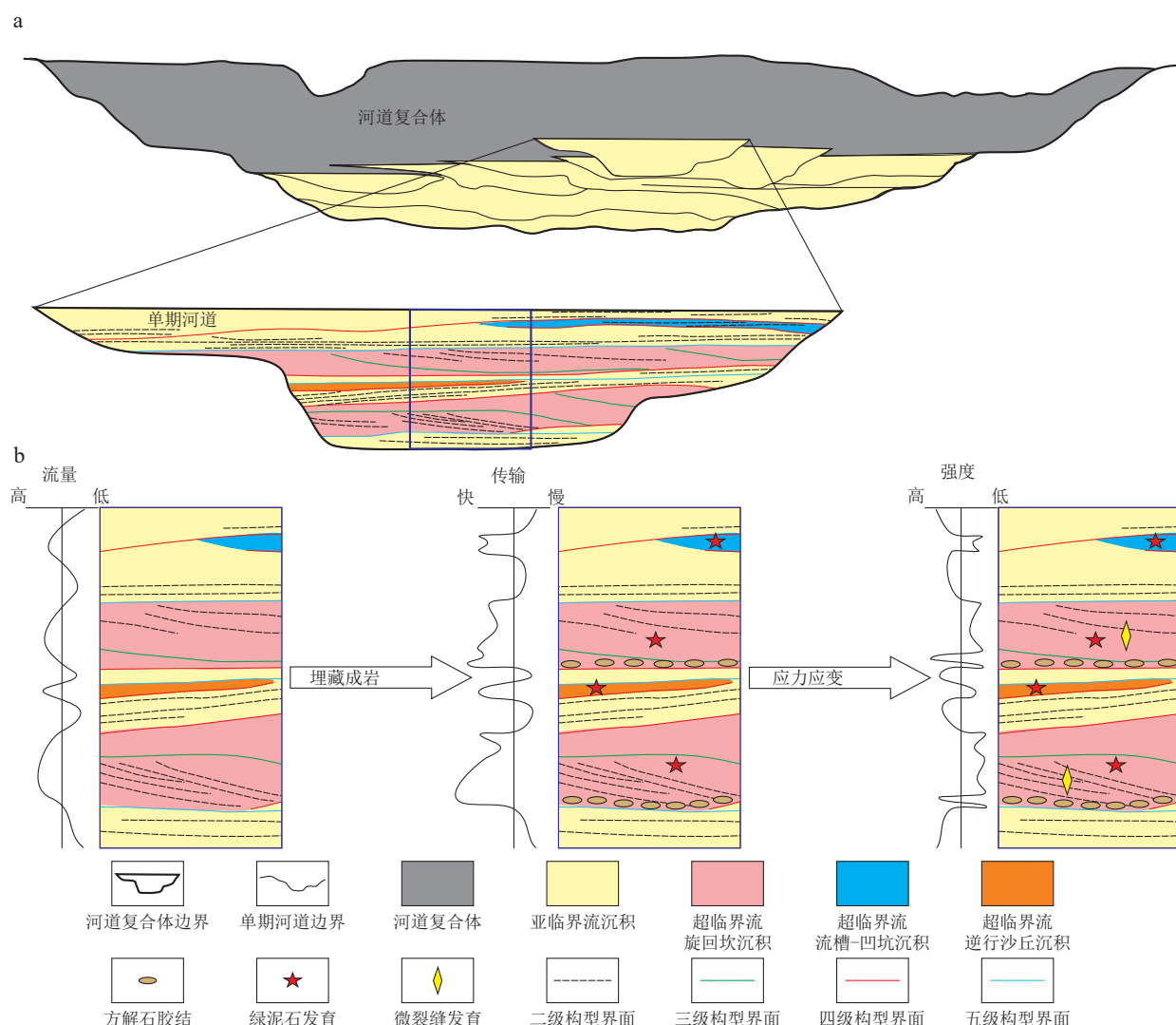
图9 四川盆地川西坳陷须二段致密碎屑岩储层“沉积-成岩-破裂”非均质性综合模式示意图(据文献[23]修改)
