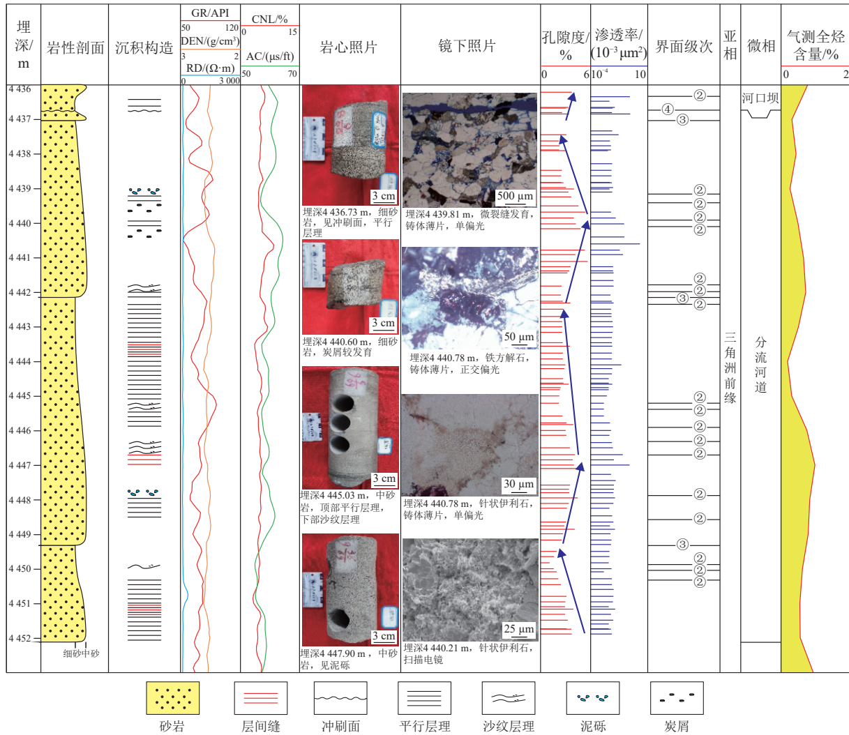
图6 四川盆地川西坳陷川丰563井须二段1砂组致密碎屑岩储层非均质性特征
