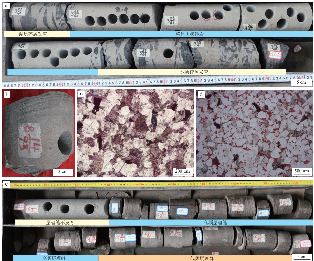
图5 四川盆地川西坳陷须二段致密碎屑岩储层沉积、成岩与破裂非均质性特征照片
