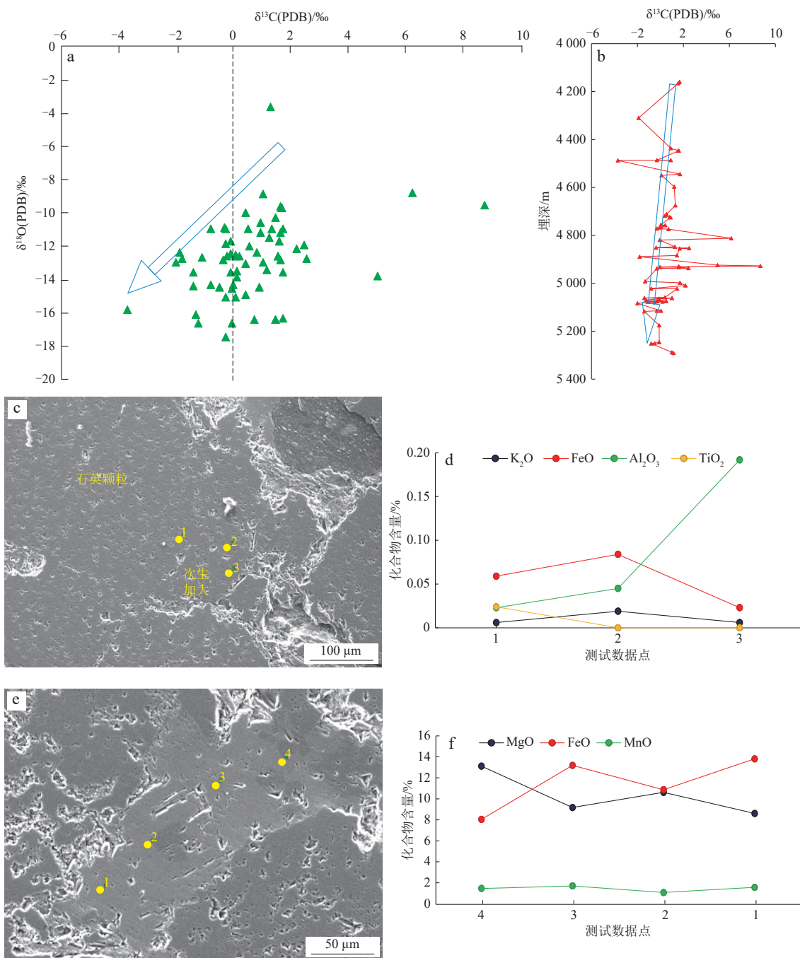
图7 四川盆地川西坳陷须二段致密碎屑岩储层胶结物形成过程中的物质迁移
