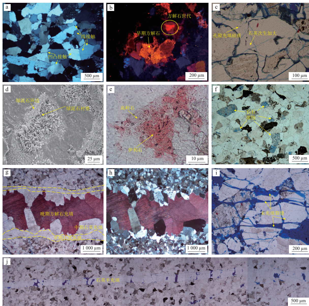
图3 四川盆地川西坳陷须二段致密碎屑岩储层成岩作用与微裂缝特征镜下照片
