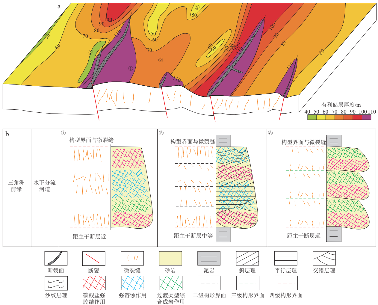
图8 四川盆地川西坳陷须二段致密碎屑岩储层不同沉积岩相组合控制的成岩作用与微裂缝发育的差异性模式示意图
