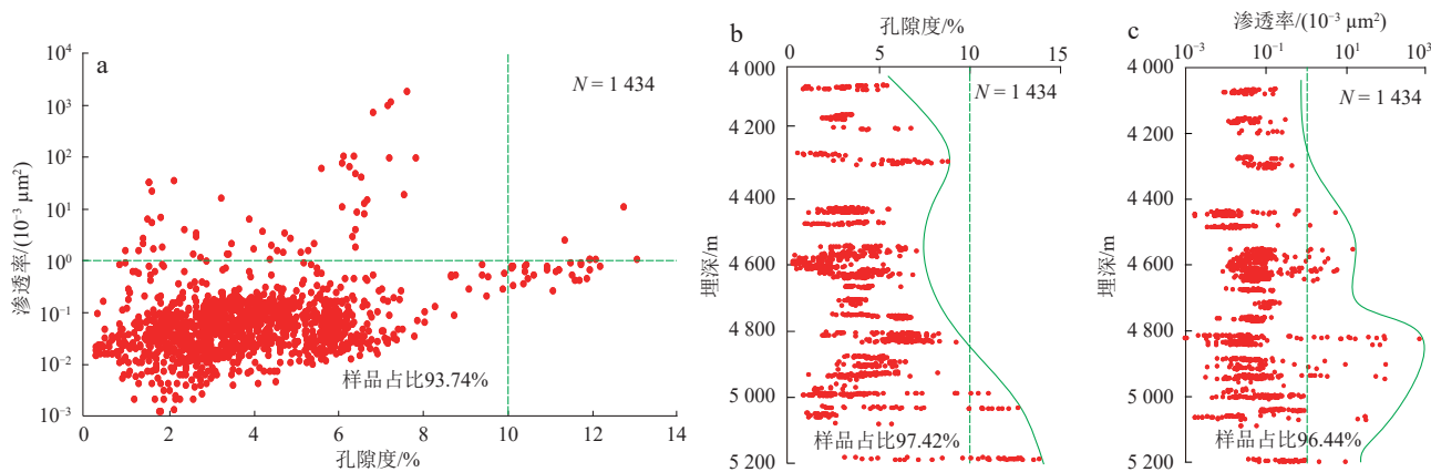
图2 四川盆地川西坳陷须二段储层物性特征
