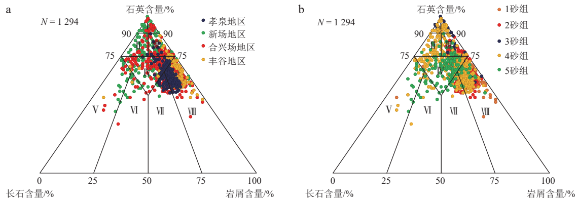
图4 四川盆地川西坳陷须二段致密碎屑岩储层岩石学特征三角图
