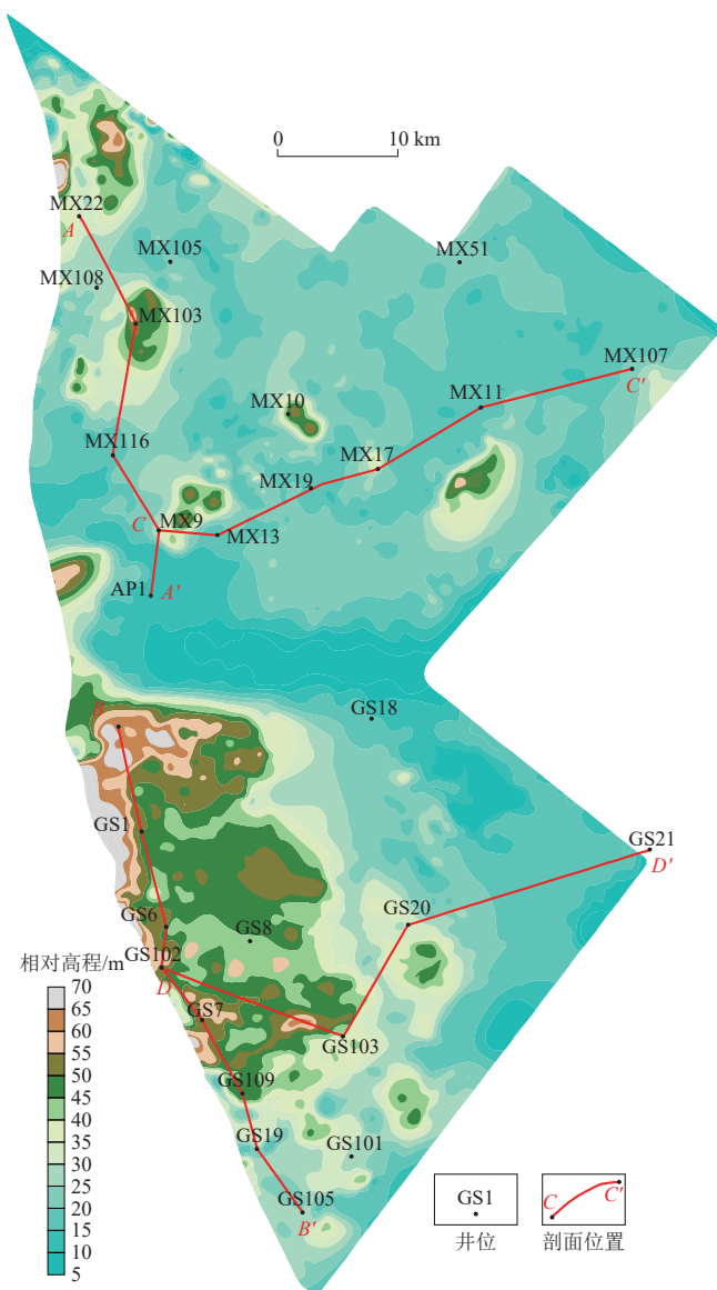
图8 四川盆地高磨地区灯四段沉积古地貌
