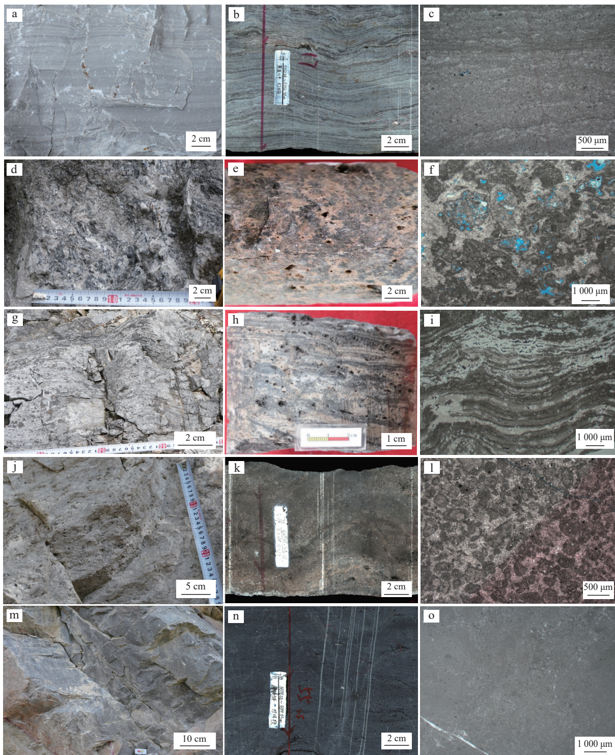
图2 四川盆地灯四段丘滩沉积微相典型露头、岩心及薄片特征照片
