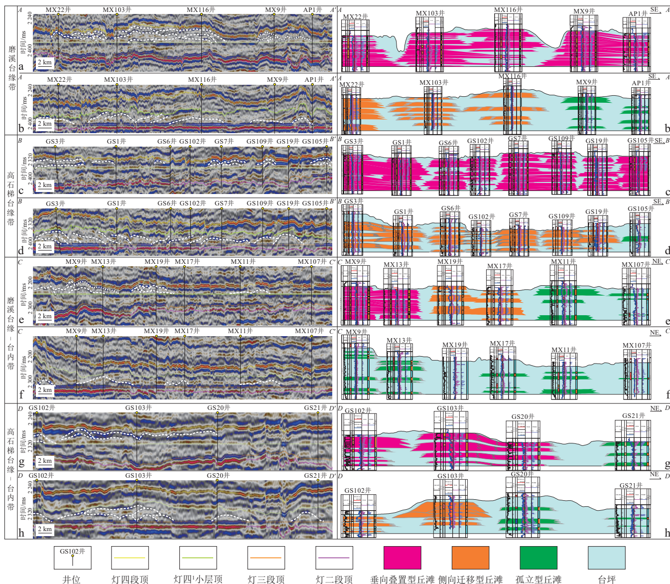
图12 四川盆地高磨地区灯四段丘滩叠置样式地震剖面(a—h)及连井剖面(a'—h')(剖面位置见图8)
