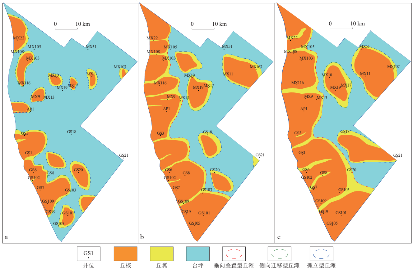
图11 四川盆地高磨地区灯四段各小层丘滩平面分布
