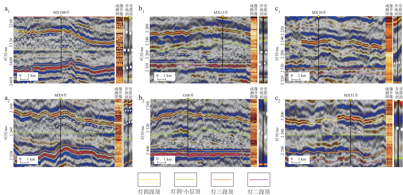
图5 四川盆地高磨地区灯四段不同叠置样式丘滩地震剖面特征
