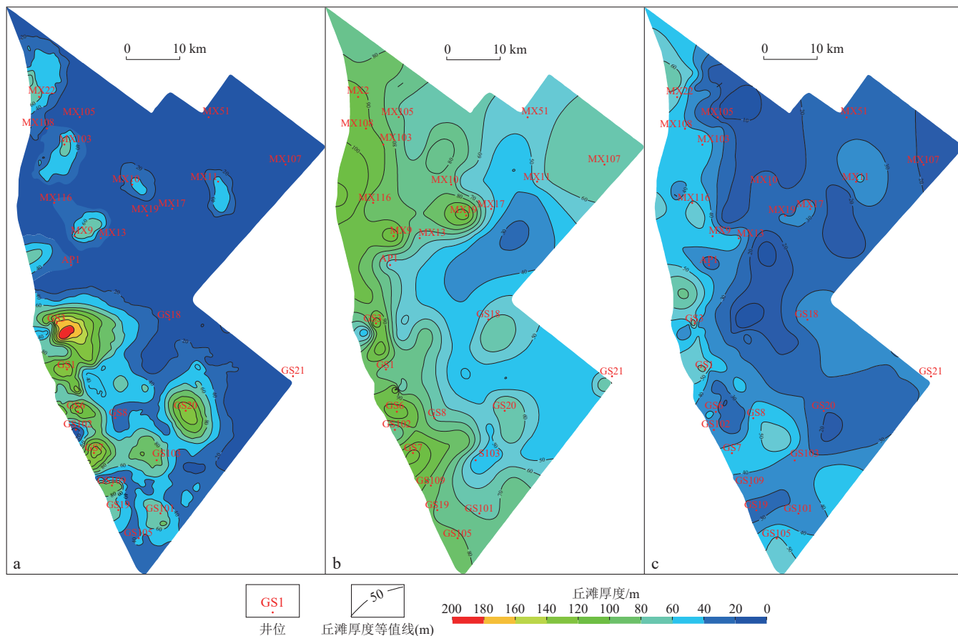
图9 四川盆地高磨地区灯四段各小层丘滩厚度平面分布等值线图
