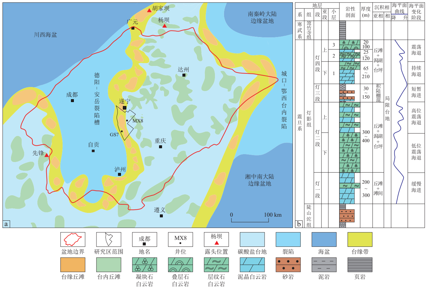
图1 四川盆地晚震旦世构造及沉积特征
