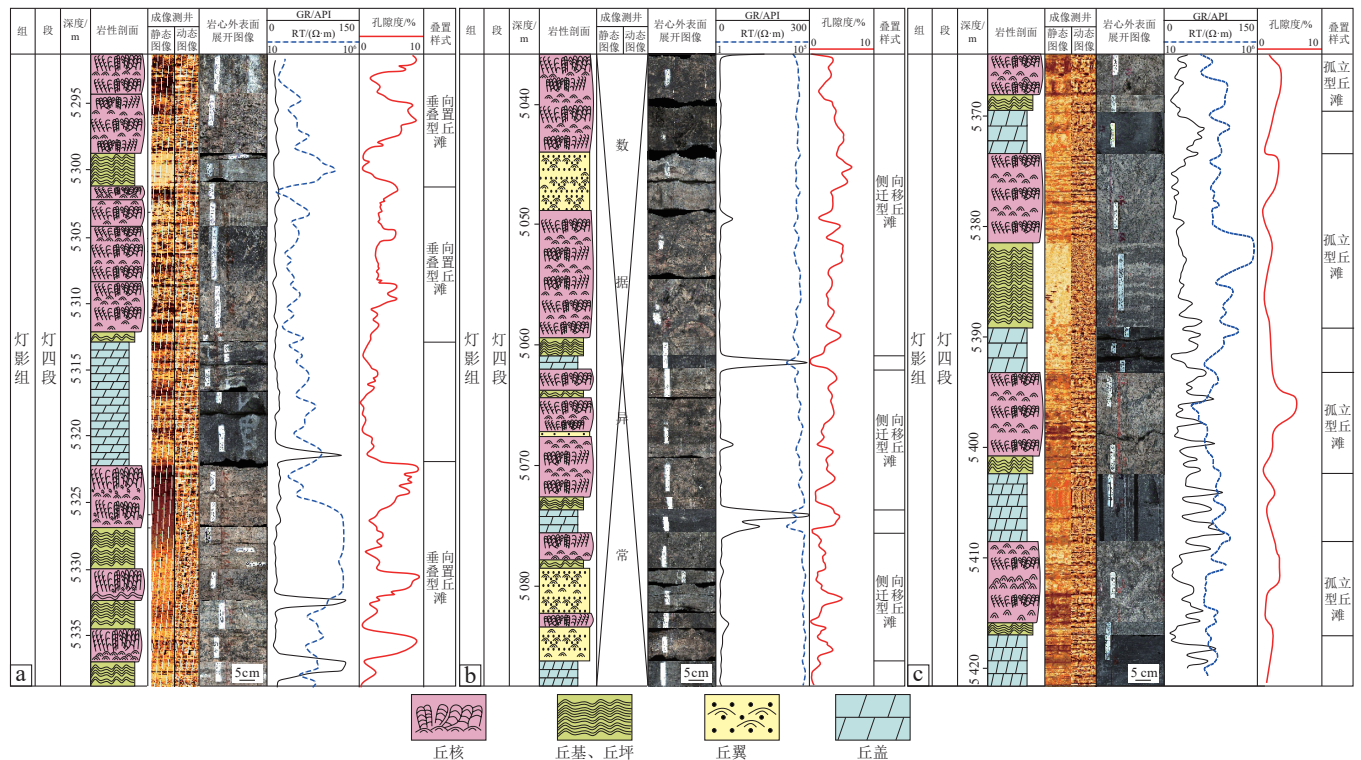
图4 四川盆地高磨地区灯四段不同叠置样式丘滩岩性组合特征
