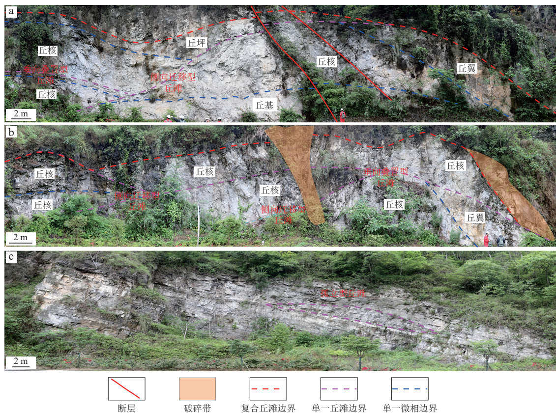
图6 四川盆地峨边先锋剖面灯影组不同叠置样式丘滩露头特征野外照片
