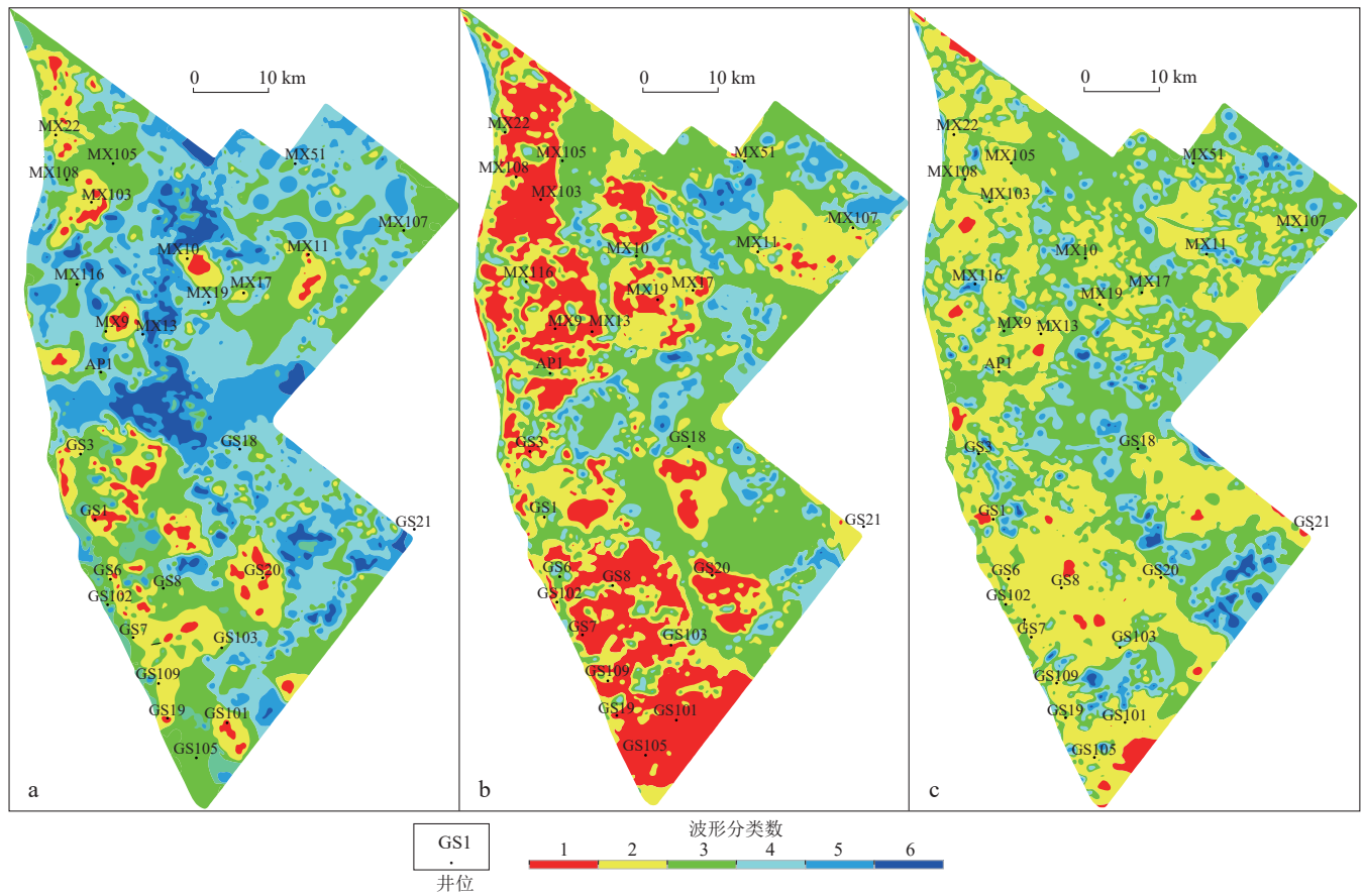
图10 四川盆地高磨地区灯四段各小层地震波形平面分布
