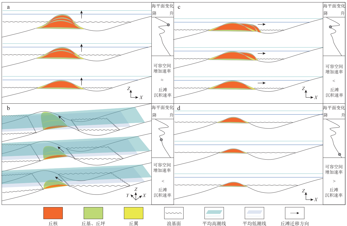
图7 四川盆地高磨地区灯四段不同叠置样式丘滩发育模式示意图
