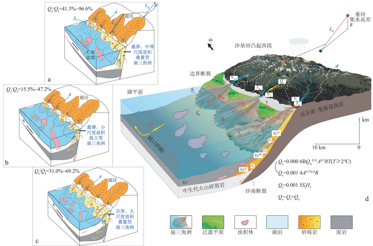
图9 渤海湾盆地沙垒田凸起西段沙三段陡坡带完整裂陷幕不同层序单元源-汇配置关系(a—c, E_s^{3L} \sim E_s^{3U} )及耦合沉积层序模式(d)
