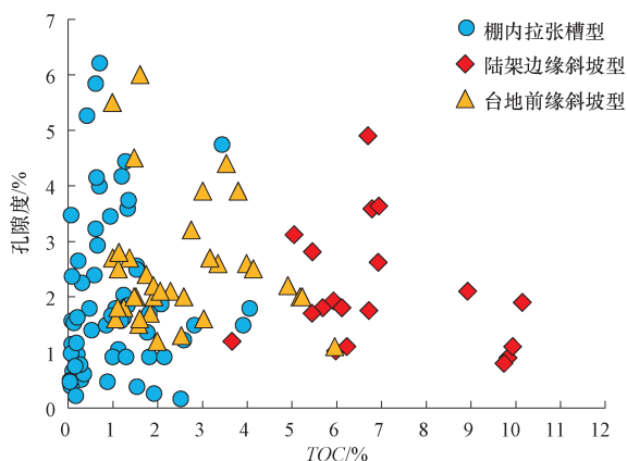
图 10 中上扬子地区下寒武统页岩 TOC 与孔隙度关系
