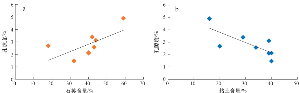
图9 中上扬子地区下寒武统陆架边缘斜坡型页岩矿物含量与孔隙度关系
