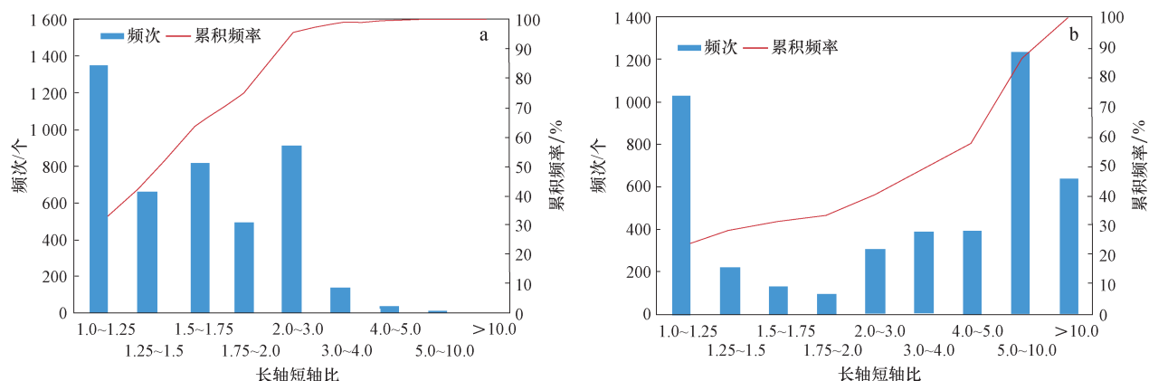
图7 中上扬子地区下寒武统不同类型页岩有机质孔长轴/短轴比特征
