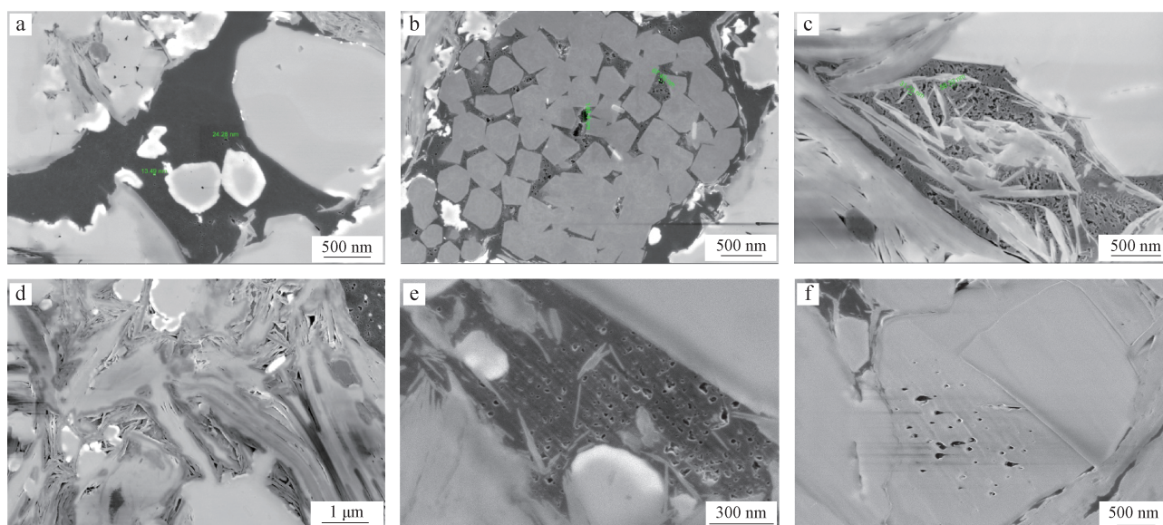
图5 中上扬子地区下寒武统不同类型富有机质页岩孔隙镜下特征
