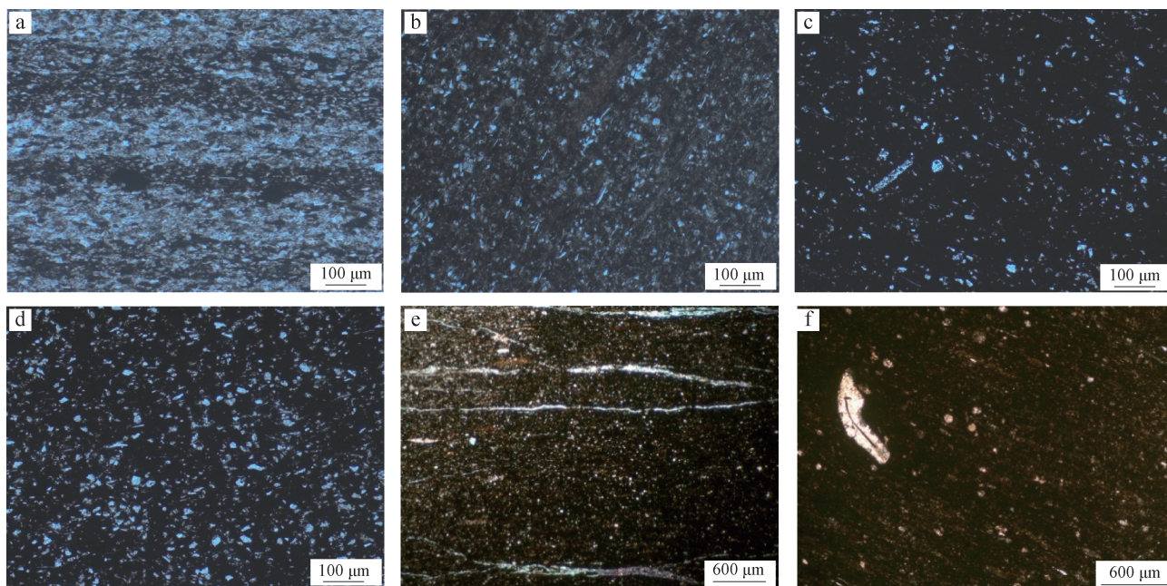
图4 中上扬子地区下寒武统不同类型富有机质页岩岩石薄片镜下特征
