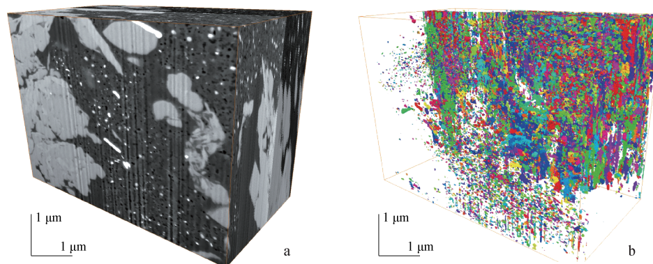
图6 中上扬子地区下寒武统陆架边缘斜坡型富有机质页岩三维孔隙结构特征
