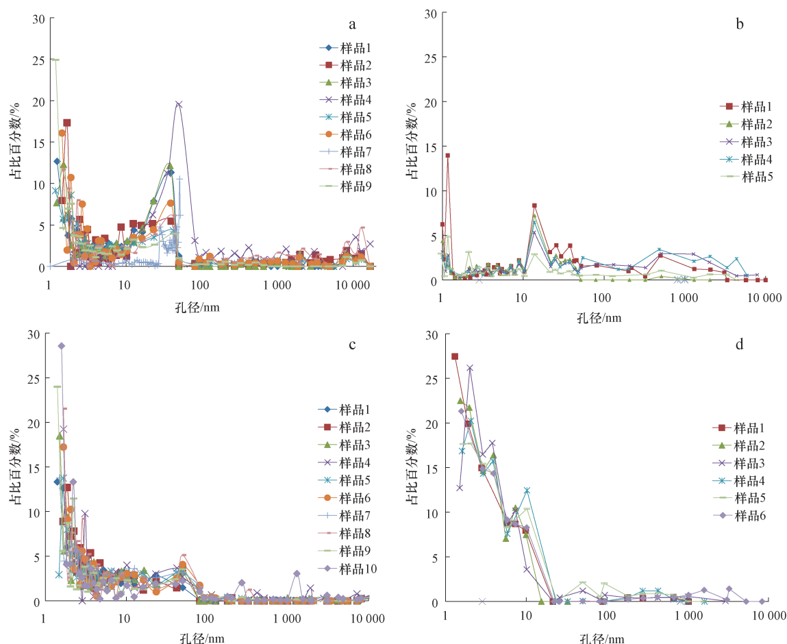
图8 中上扬子地区下寒武统页岩高压压汞-氮气吸附联合测定孔隙结构特征
