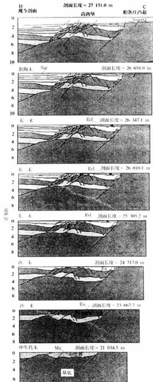
图5 南堡凹陷高尚堡构造带剖面构造恢复
