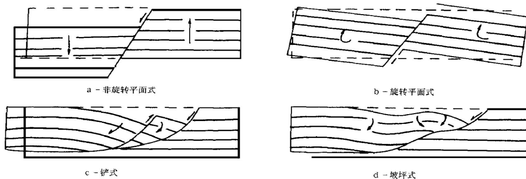
图4 正断层的几何学和运动学特征分类
