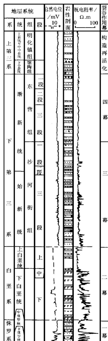
图 1 南堡凹陷幕式充填柱状图 Fig. 1 Columnar section of episodic filling in Nanpu Sag
